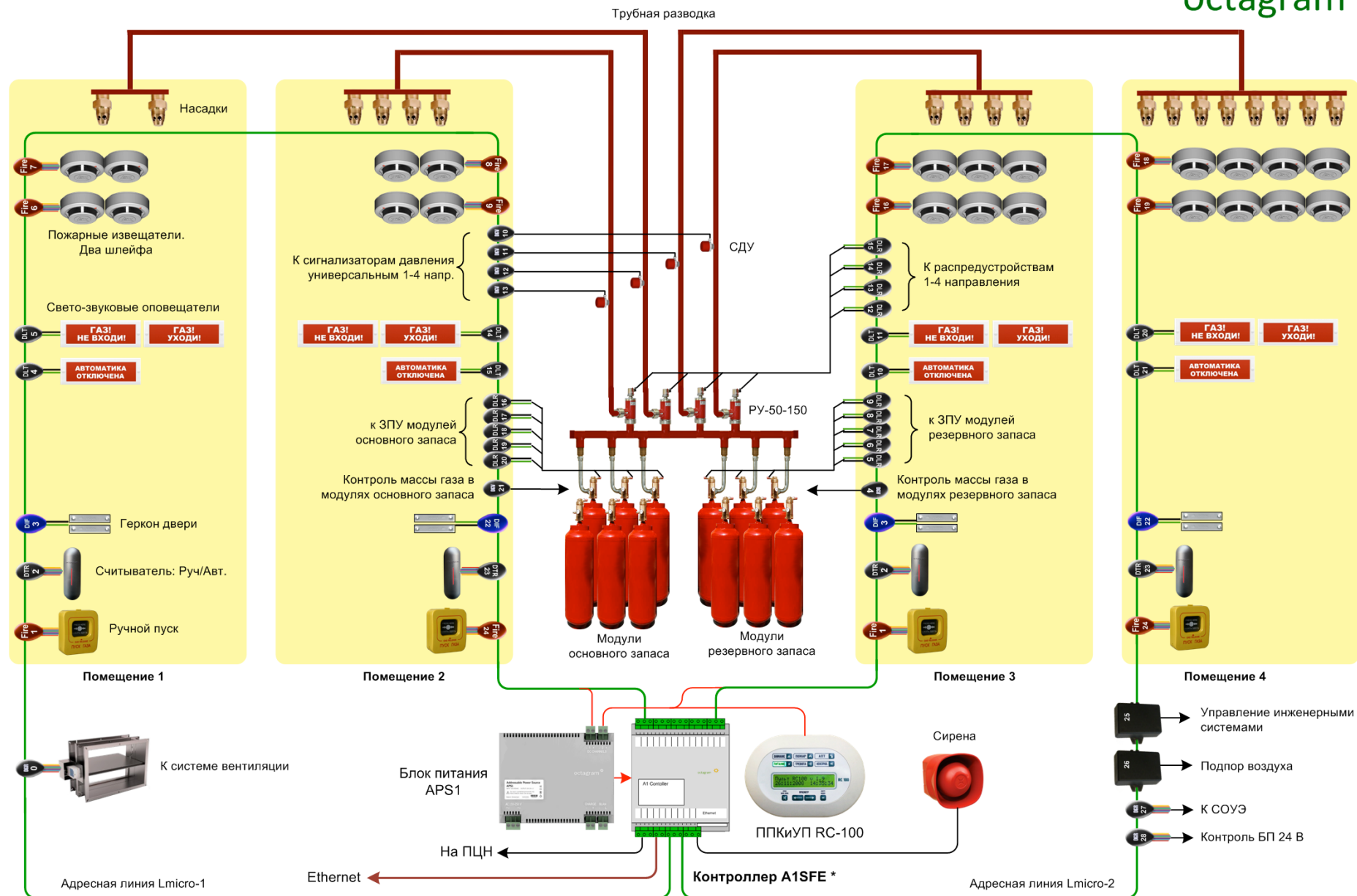
Автоматическая система газового пожаротушения (АУГП) на 4 направления
